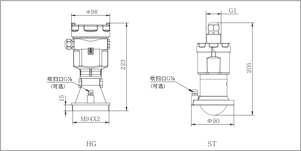
SDRD87/88 Antenna:HG/ST
